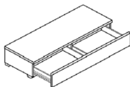
Тумба 29 см с ящиками 130 x 48 x 29 Y07-0461
